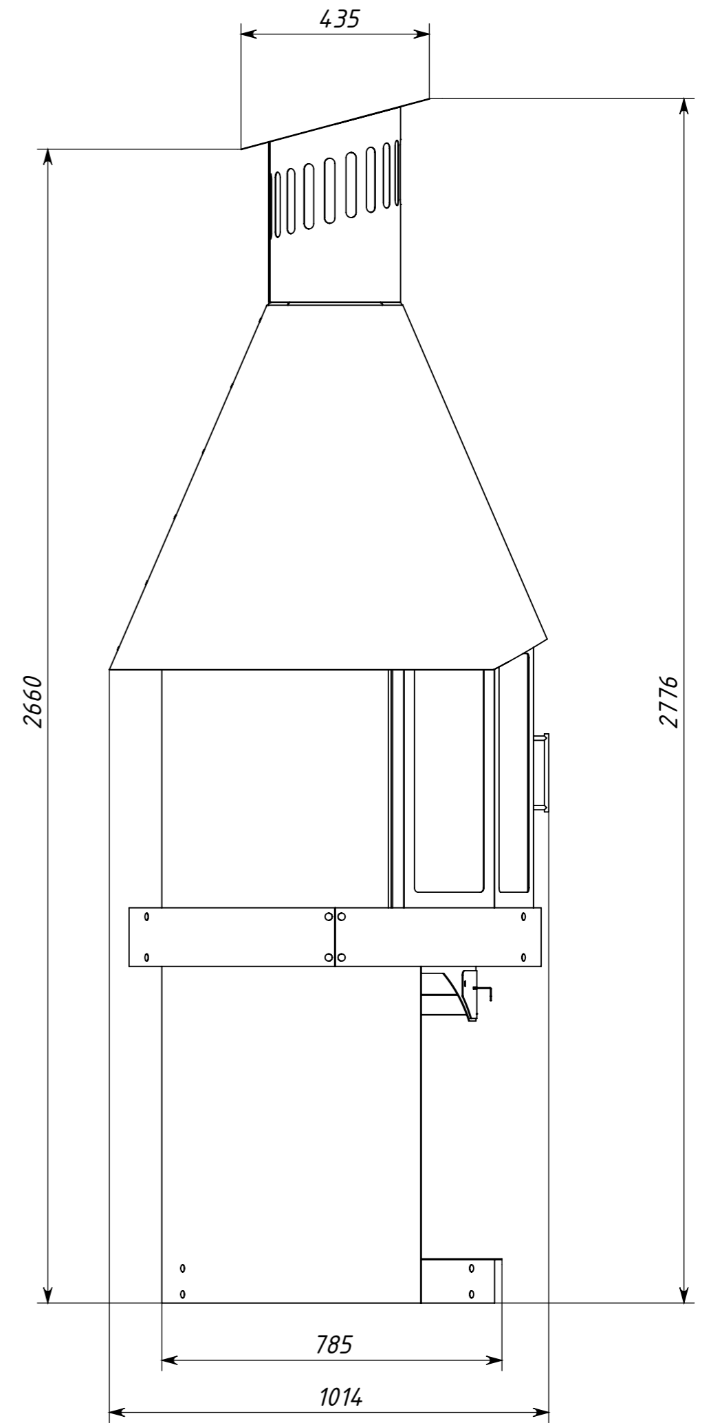
Деталь "Зонт" условно не отображена
