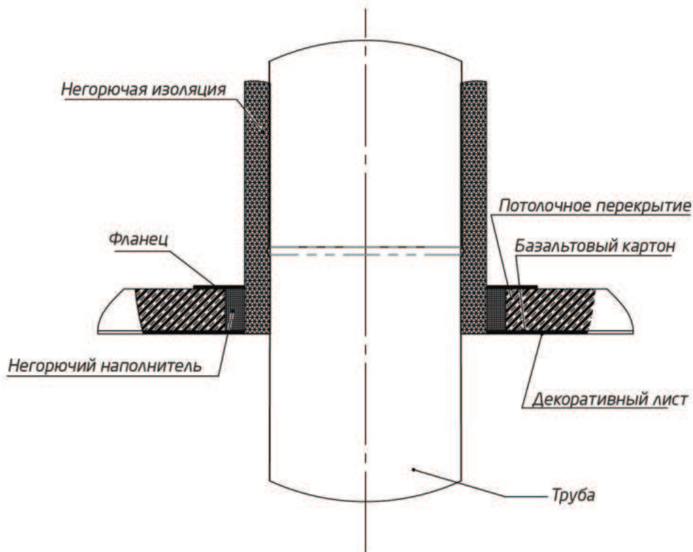
Потолочно-проходной узел
