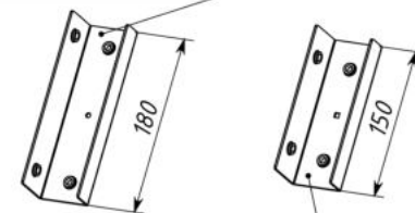
7 Профиль соединительный, верхний, 4 шт.
